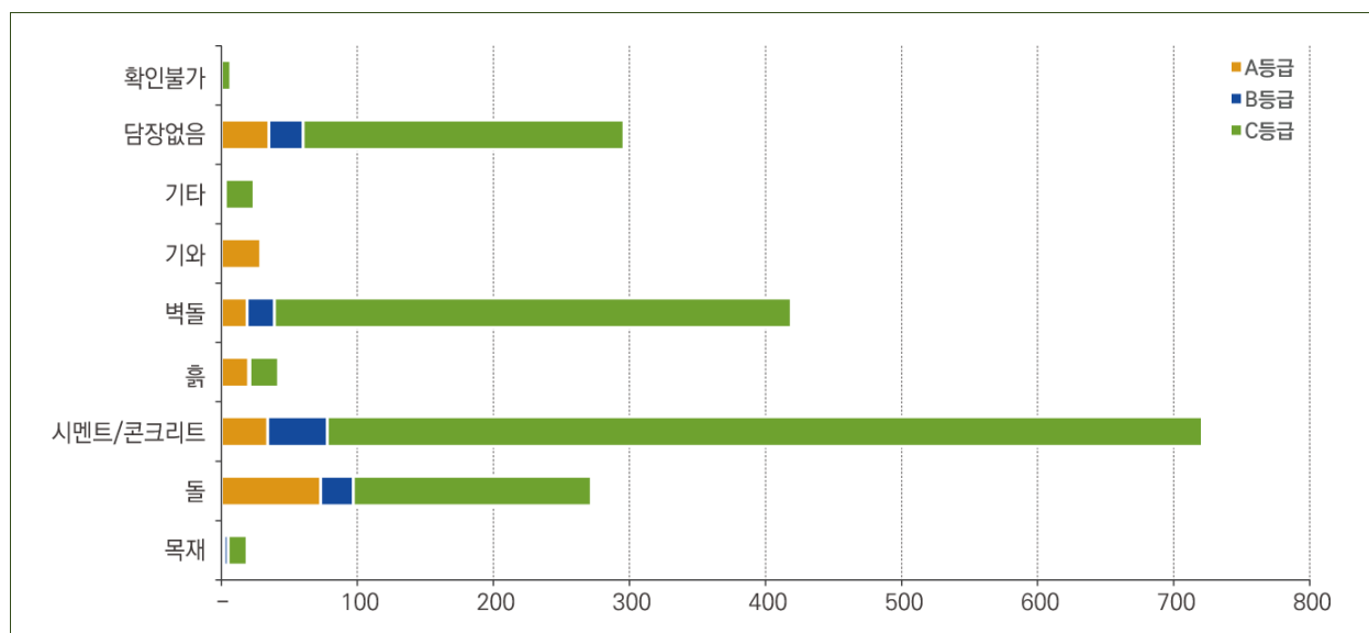
[경상북도 포항시 북구 담장재료별 한옥현황]
