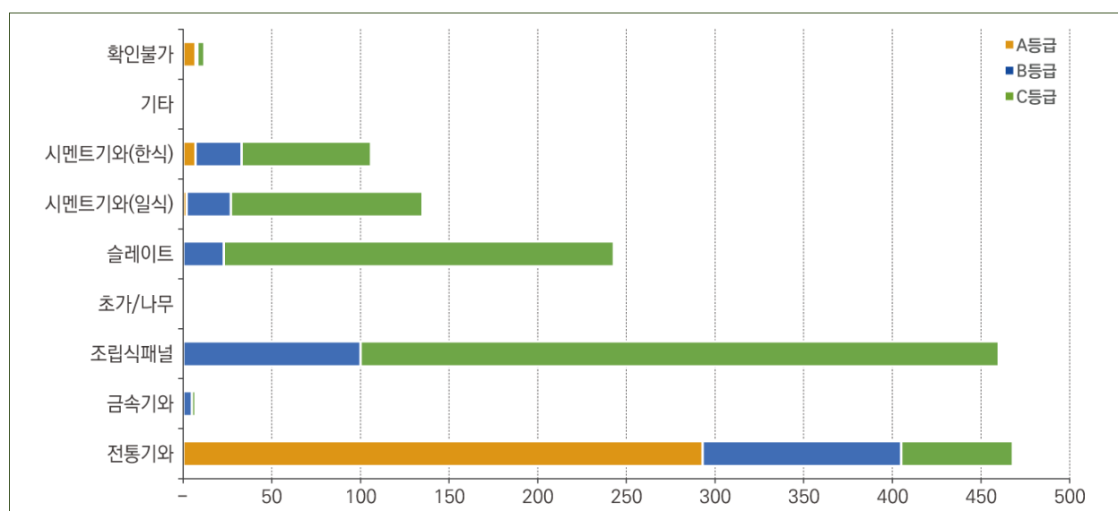
[경상북도 청도군 지붕재료별 한옥현황]
