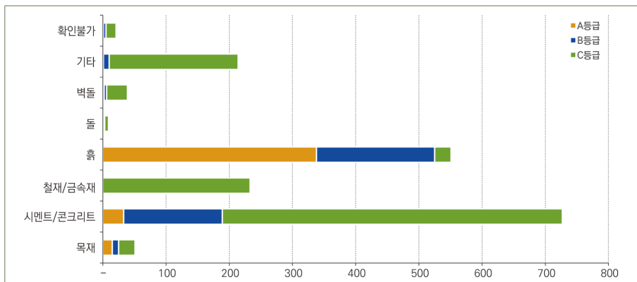
[경상북도 청송군 외벽재료별 한옥현황]
