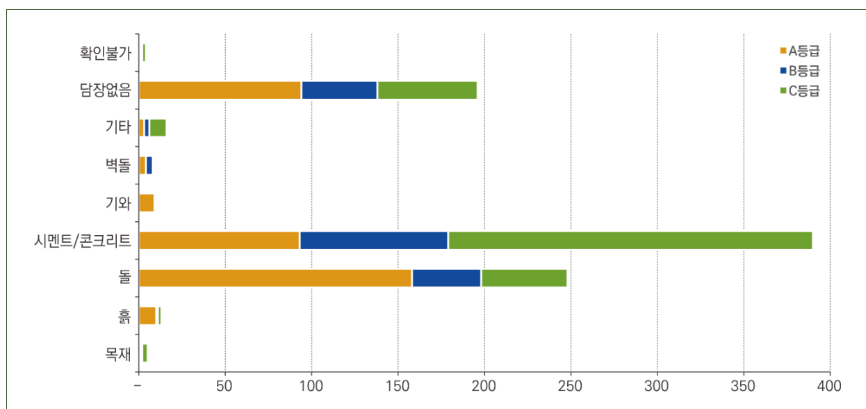
[경상북도 칠곡군 담장재료별 한옥현황]
