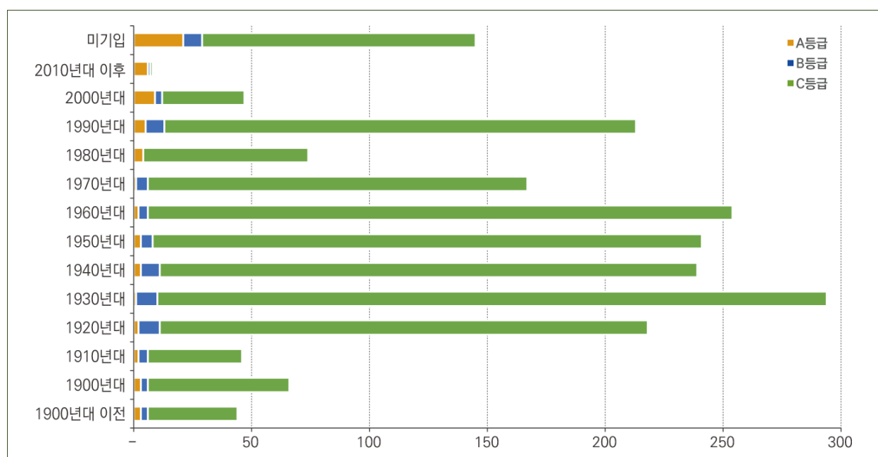
[경상북도 울진군 건축시기별 한옥현황]
