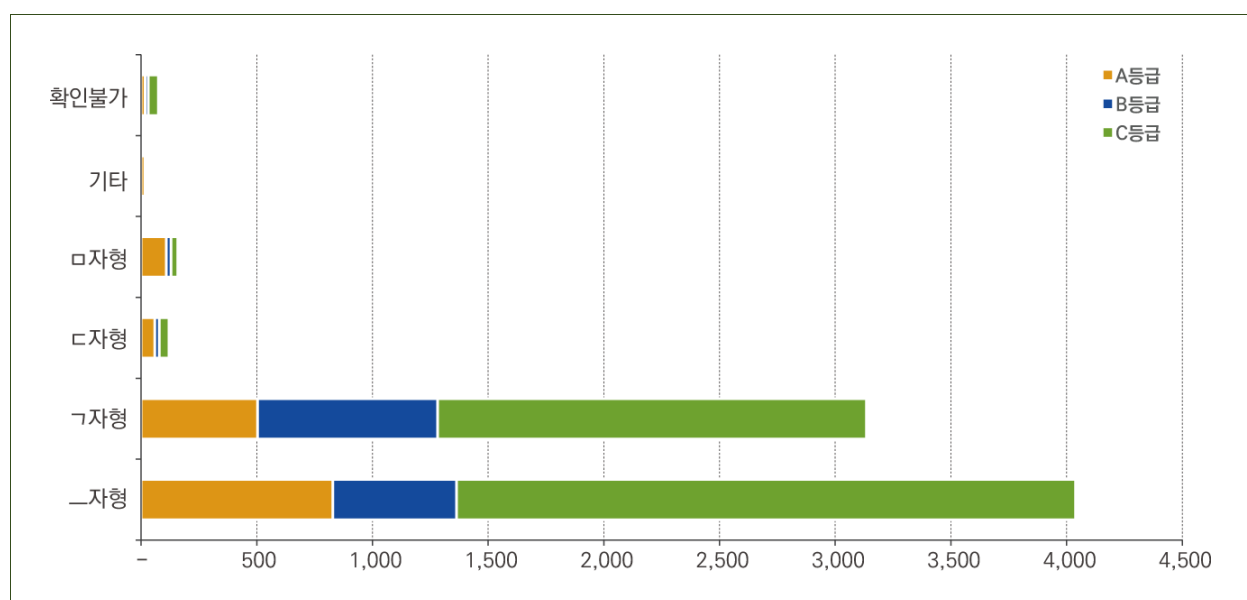
[경상북도 안동시 평면형태별 한옥현황]
