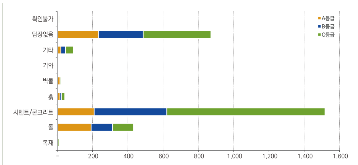
[경상북도 의성군 담장재료별 한옥현황]
