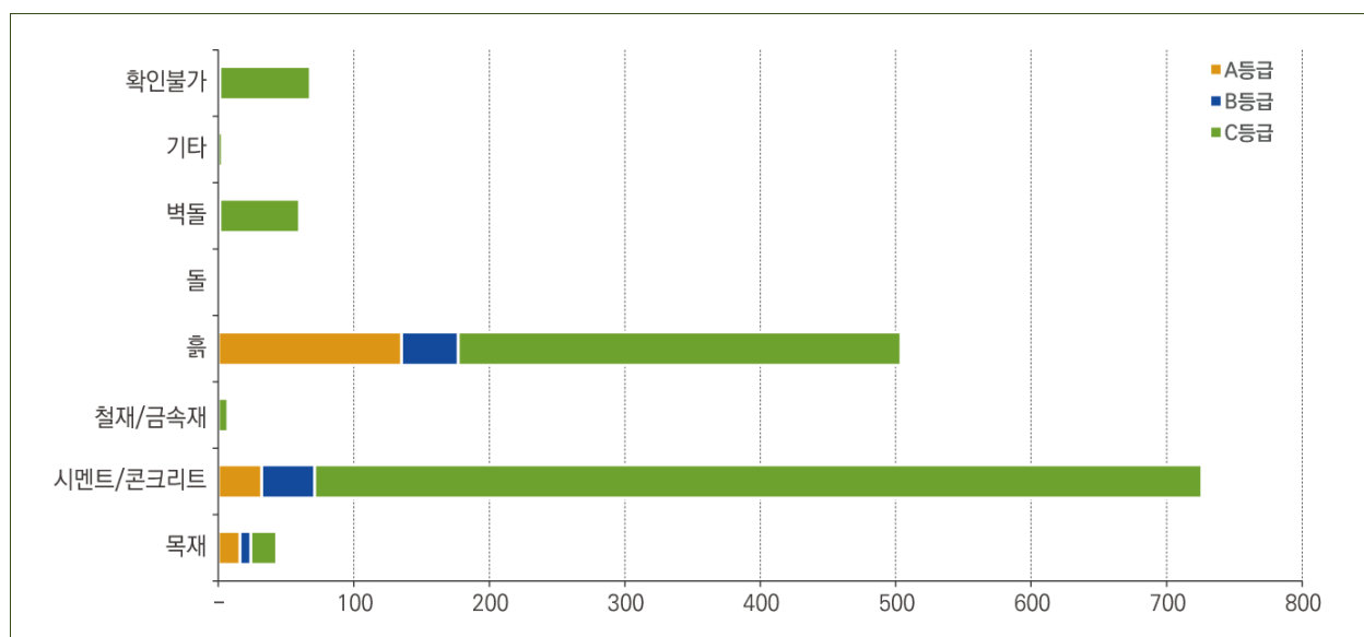
[경상북도 경산시 외벽재료별 한옥현황]
