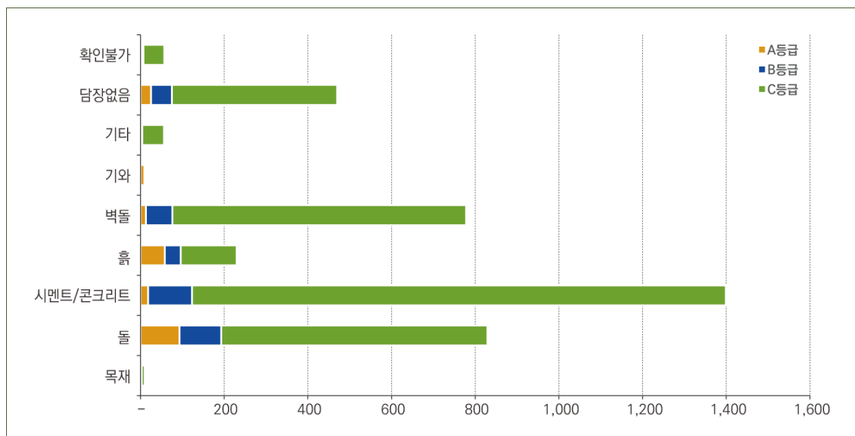
[경상북도 고령군 담장재료별 한옥현황]
