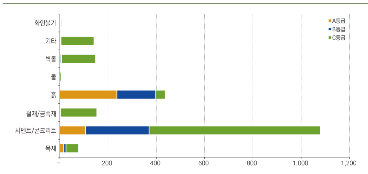
[경상북도 영양군 외벽재료별 한옥현황]
