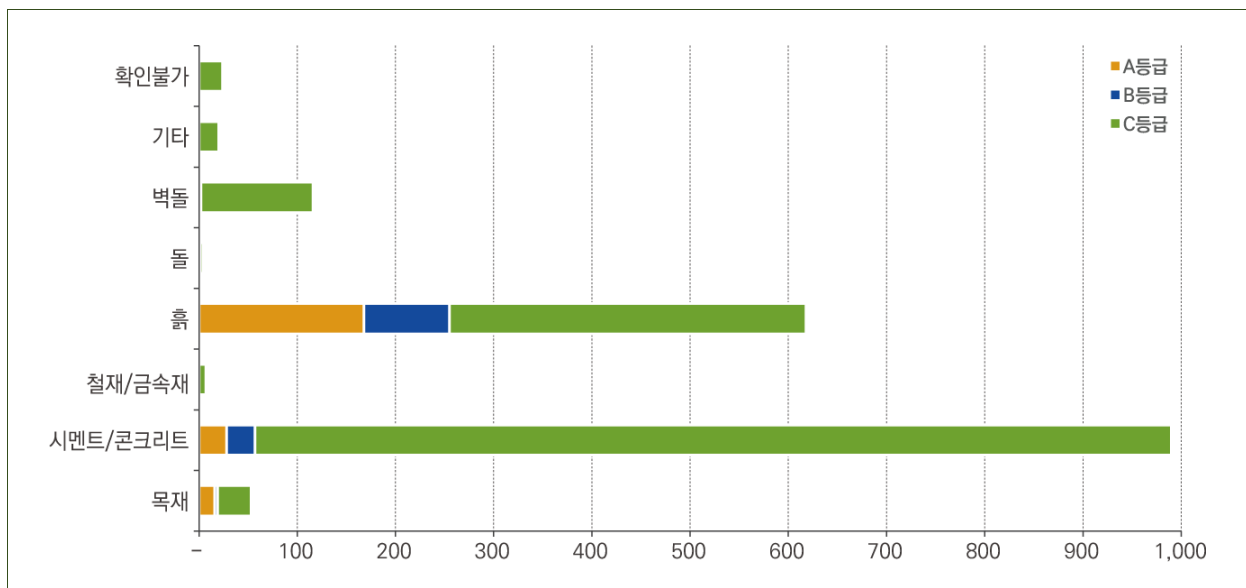
[경상북도 포항시 북구 외벽재료별 한옥현황]
