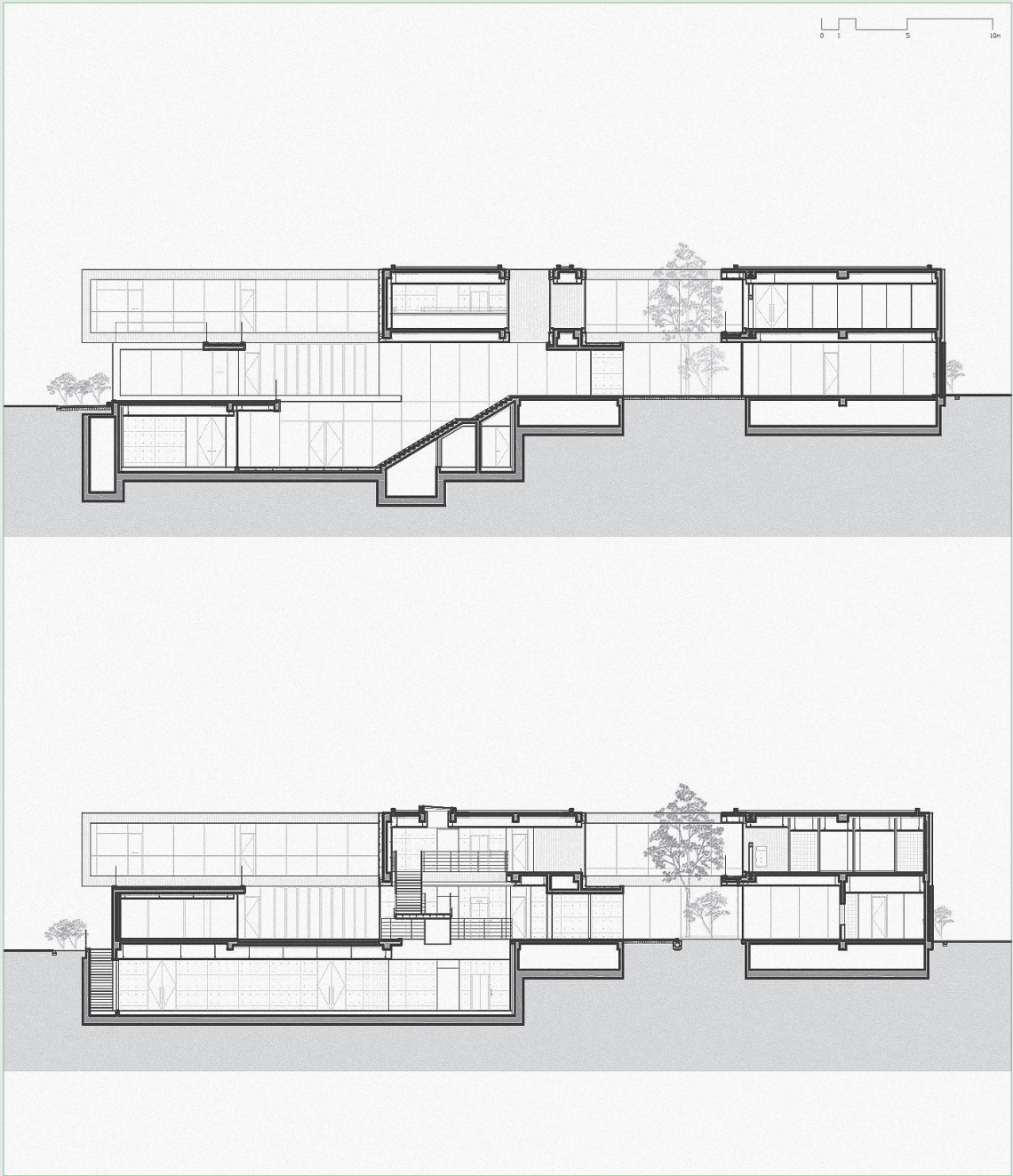
횡단면도
